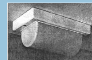
Giso no. 813 (1 stuks). Gisocatalogus no. 29, pagina 80. Waterdichte plafonnier porselein. Hoogte 6,5 cm. Voor gloeilampen tot 75 watt.
